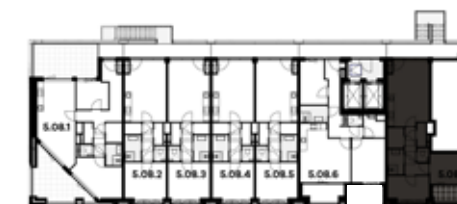
4 E VERDIEPING
