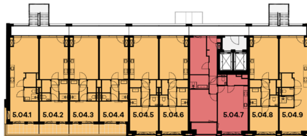
VIERDE VERDIEPING
