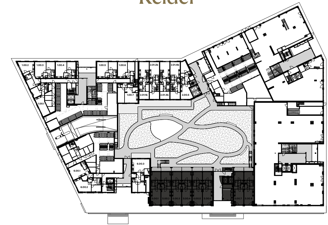
Begane grond
