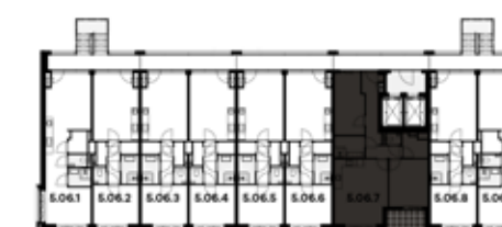
6 E VERDIEPING
