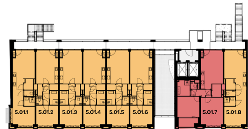
EERSTE VERDIEPING
