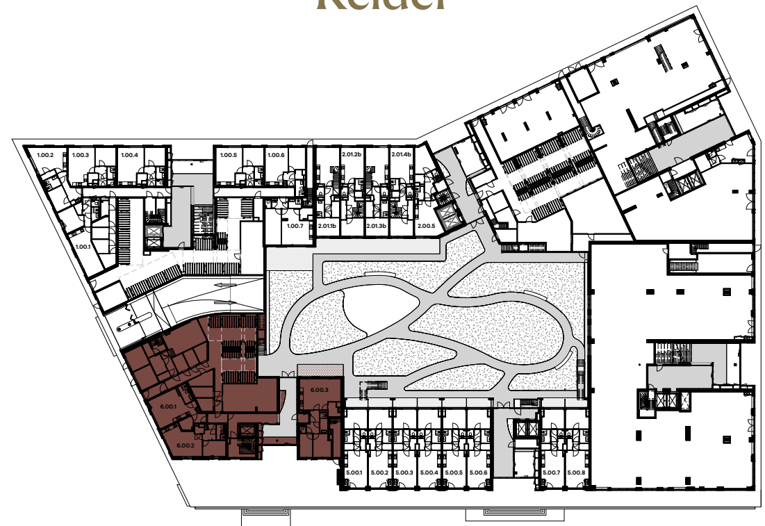
Begane grond
